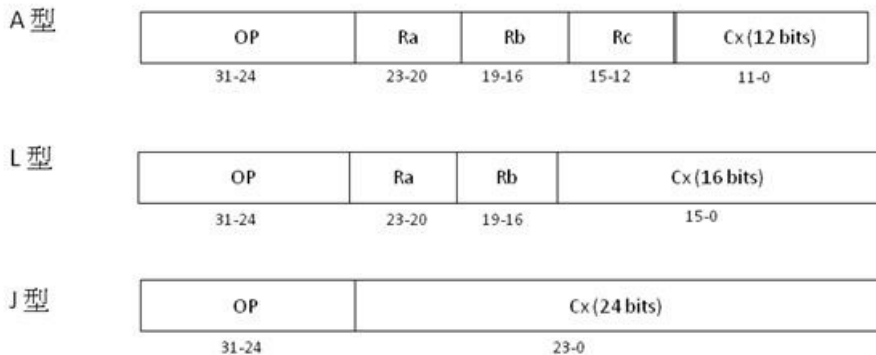
圖、CPU0的指令格式
